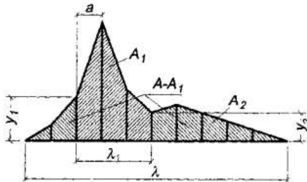
Рисунок Б.2 – Частина лінії впливу завдовжки \lambda , що включає її вершину
