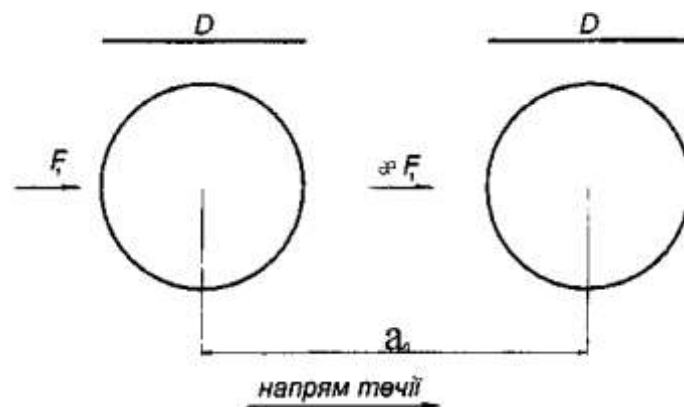
Рисунок К.1 – Схема до розрахунку тиску при прорізуванні льоду опорами
