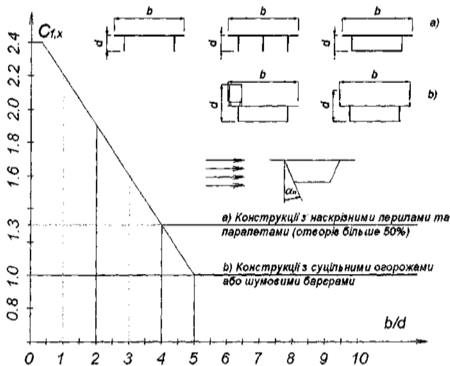
Рисунок Л.1 – Графік зміни коефіцієнта C_{f,x}
