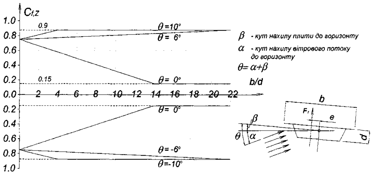
Рисунок Л.2 – Графік зміни коефіцієнта C_{f,z}
