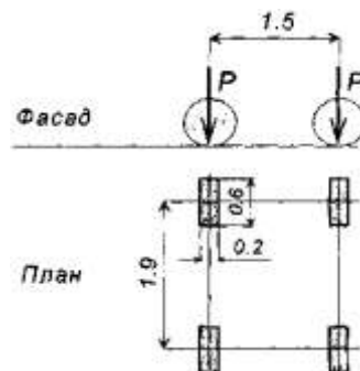
Рисунок 18.1 – Схема навантаження тандема АК
