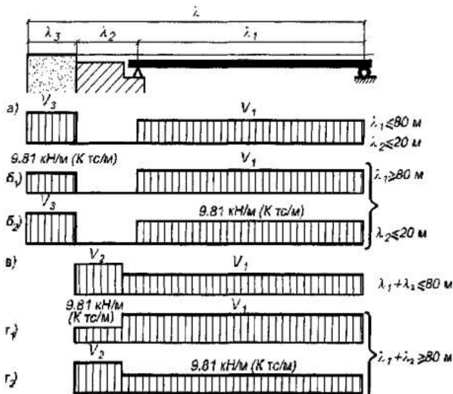
Рисунок Б.3 – Схема завантаження ділянок лінії впливу при \lambda > 80 м
