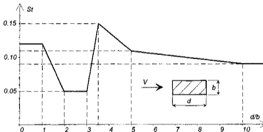
Рисунок Л.2.1 – Значення числа Струхалія для прямокутного тіла
