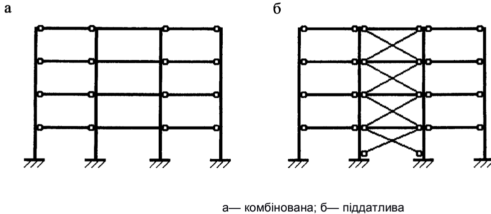
Рисунок 3 - Схеми рам каркасів багатопверхових будинків
