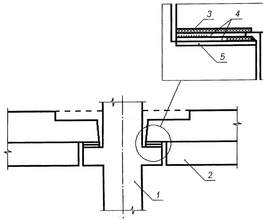
1 - колона; 2 - шарнірно-обпертий ригель; 3 - закладна деталь ригеля; 4 - нижня і верхня зв'язкові пластини; 5 - закладна деталь колони
