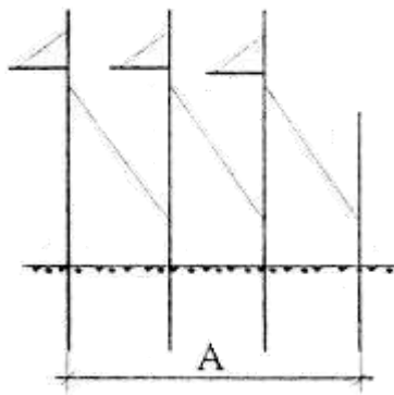
Рисунок В.6. Портальна опора з відтяжками
