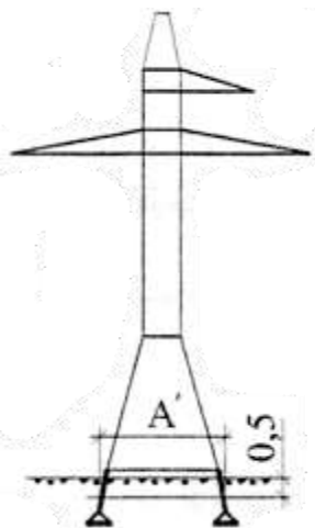
Рисунок Б.14. Баштова опора на фундаментах з вертикальними стояками
