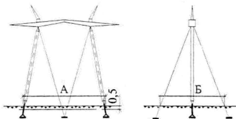
Рисунок В.5. Стояк одиночний з підтяжками в різних площинах
