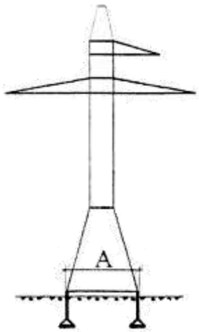
а) Схема конструкції опори
